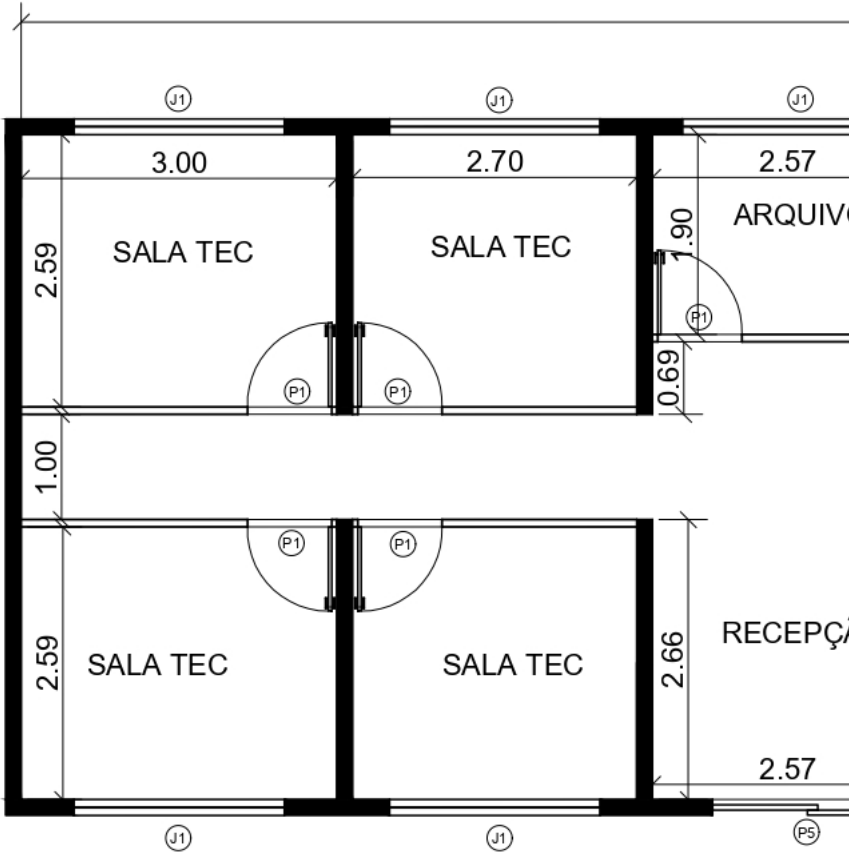
PLANTA BAIXA EXECUTIVA ESC 1: 75
