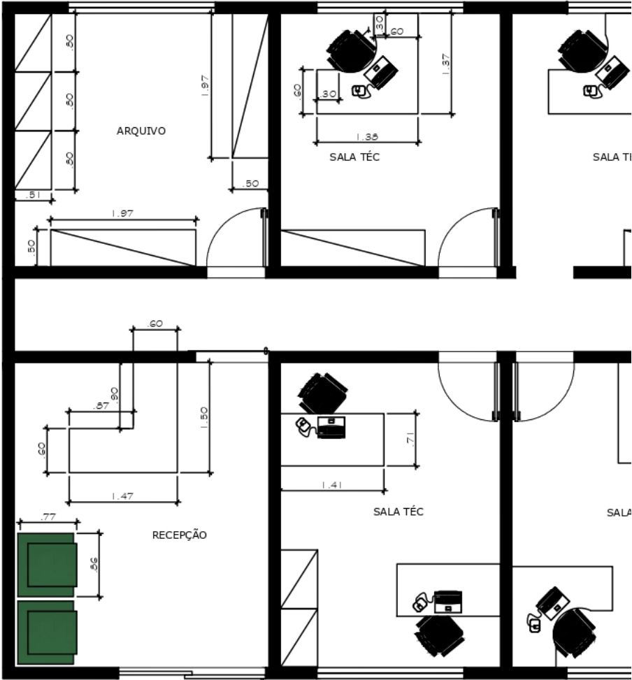
LAY OUT – MEDIDAS MOBILIÁRIO ESC 1: 75
