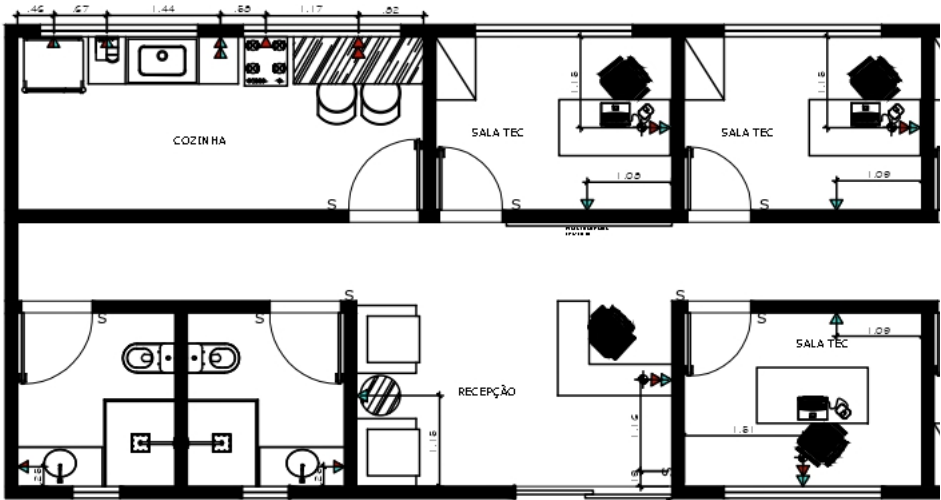
PLANTA BAIXA EXECUTIVA ESC 1:100
